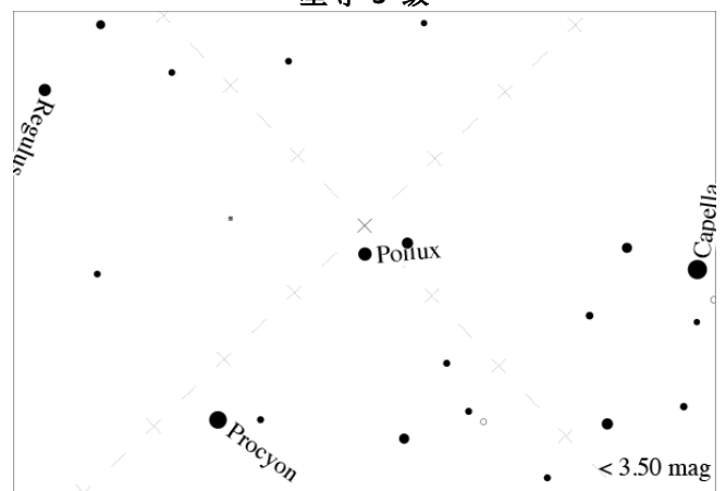
星等 3 级
